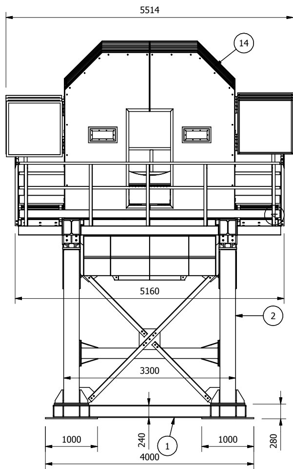
VISTA LATO DI SCARICO
